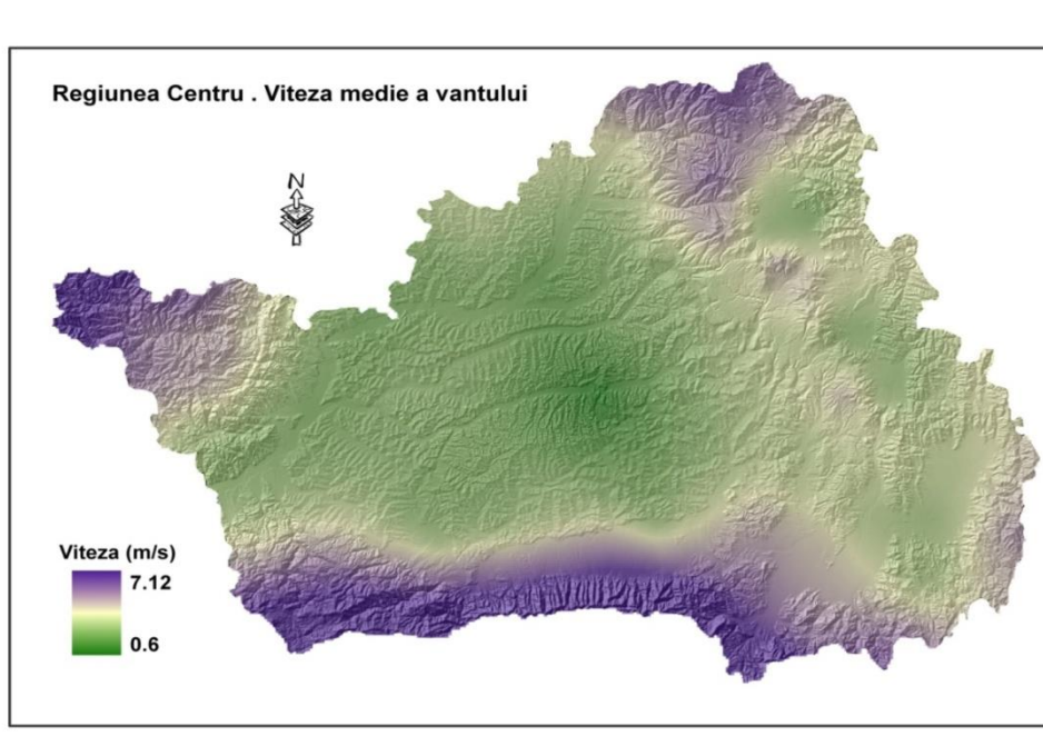
Fig. 2.4. Harta vitezelor medii anuale ale vântului în Regiunea Centru
