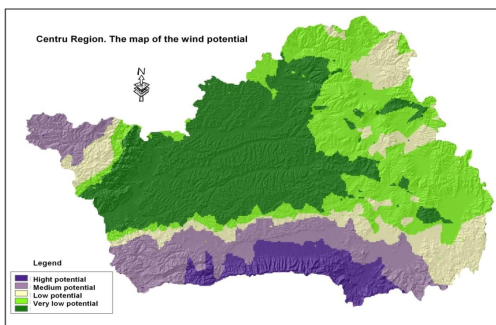
Fig. 2.5. Harta potențialului energetic eolian în Regiunea Centru
