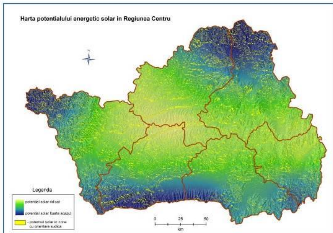
Fig. 2.2. Harta potențialului solar la nivelul Regiunii Centru
